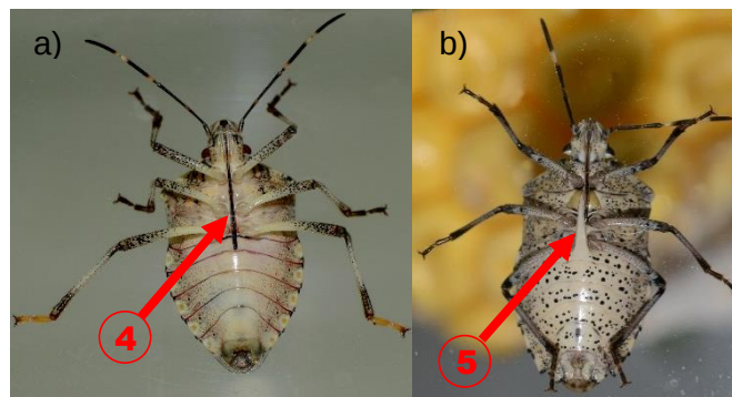
Abbildung 2 Bauchansicht a) von der Marmorierten Baumwanze, ohne Dorn zwischen den Beinen und b) von der Grauen Feldwanze mit Dorn. Foto: Tim Haye, CABI
