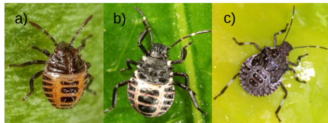
Abbildung 4 a) Nymphe im ersten, b) zweiten oder dritten und c) vierten oder fünften Stadium von H. halys .
