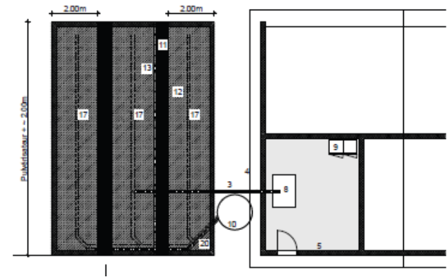
Abbildung 9: Grundriss Biobed
